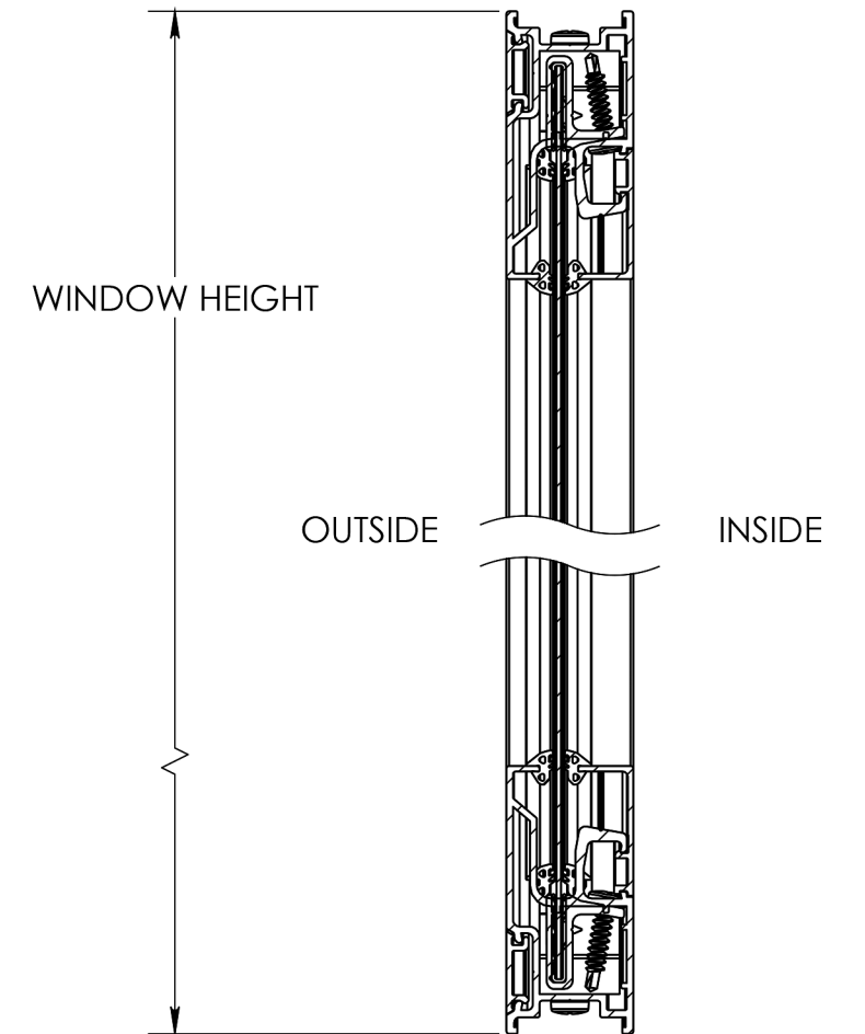
SECTION A-A
